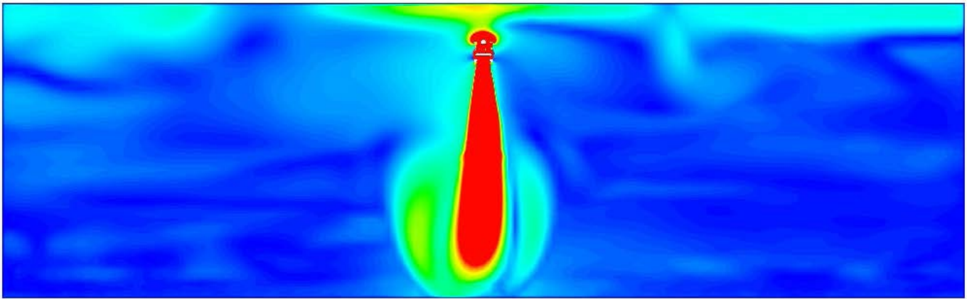
Vitesses d'air dans un plan de coupe transversal de la cellule logistique
