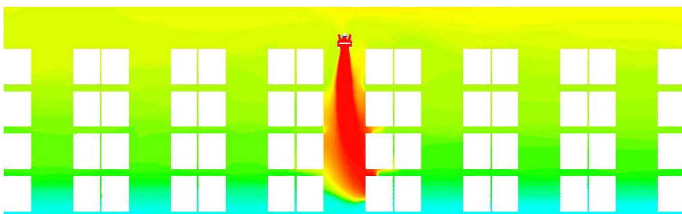
Température dans un plan de coupe transversal de la cellule logistique – Milieu de la cellule Echelle fixée [°C]
